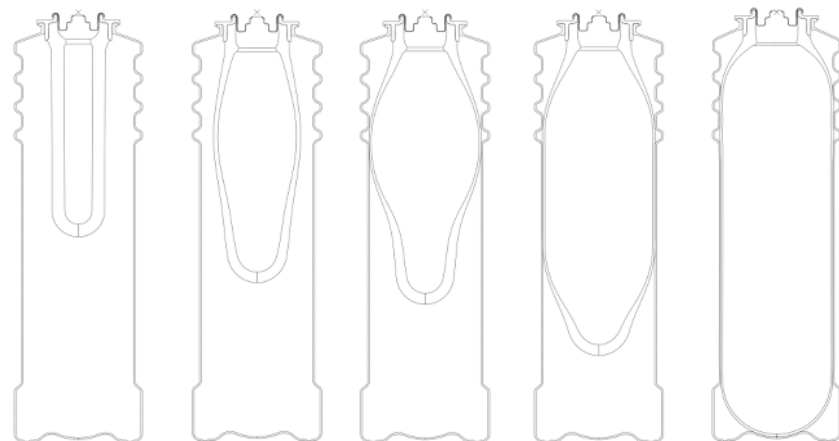
leerer Zustand
